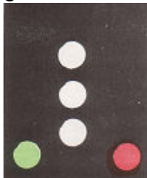
WVV slepend, duwend of langsij slepend langer of korter dan 50m, sleeplengte tot 200m inbegrepen, rechtop gezien
