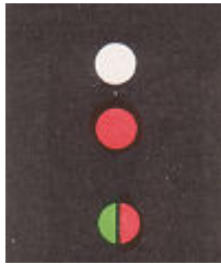
Loodsvaartuig korter dan 20m, varend, rechtop gezien
