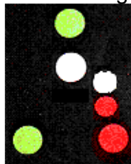
Treiler, korter dan 50m, vaartlopend, rechtop gezien, bezig met netten in te halen
