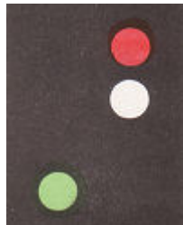
Vissersvaartuig, geen treiler, vistuig gelijk aan of korter dan 150m, vaartlopend, aan stuurboord gezien
