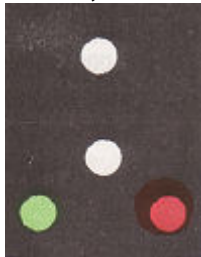
WVV langer of korter dan 50m, varend, rechtop gezien
