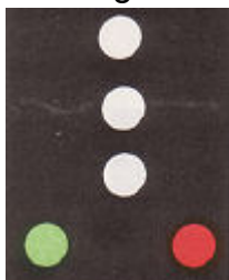
WVV slepend, korter dan 50m, sleeplengte groter dan 200m, rechtop gezien
