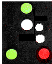
Treiler, korter dan 50m, vaartlopend, rechtop gezien, bezig met netten uit te zetten
