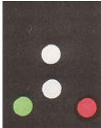
WVV slepend, duwend of langsij slepend korter dan 50m, sleeplengte tot 200m inbegrepen, rechtop gezien
