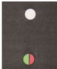
WVV korter dan 7m, max. snelheid 7kn, varend, met samengestelde lantaarn, rechtop gezien
