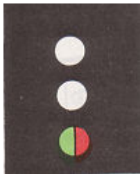
WVV slepend, duwend of langsij slepend, korter dan 20m, sleeplengte tot 200m inbegrepen, rechtop gezien, met samengestelde lantaarn
